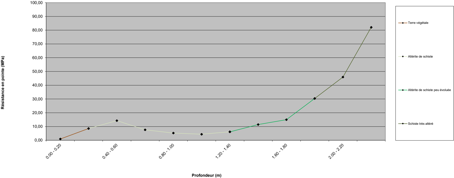
Sondage au pénétromètre dynamique - PD2 - cote NGF : 24,53 m
