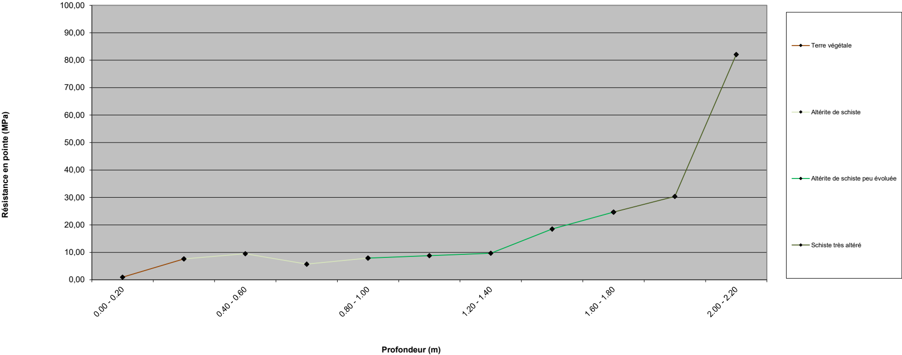
Sondage au pénétromètre dynamique - PD1 - cote NGF : 23,86 m
