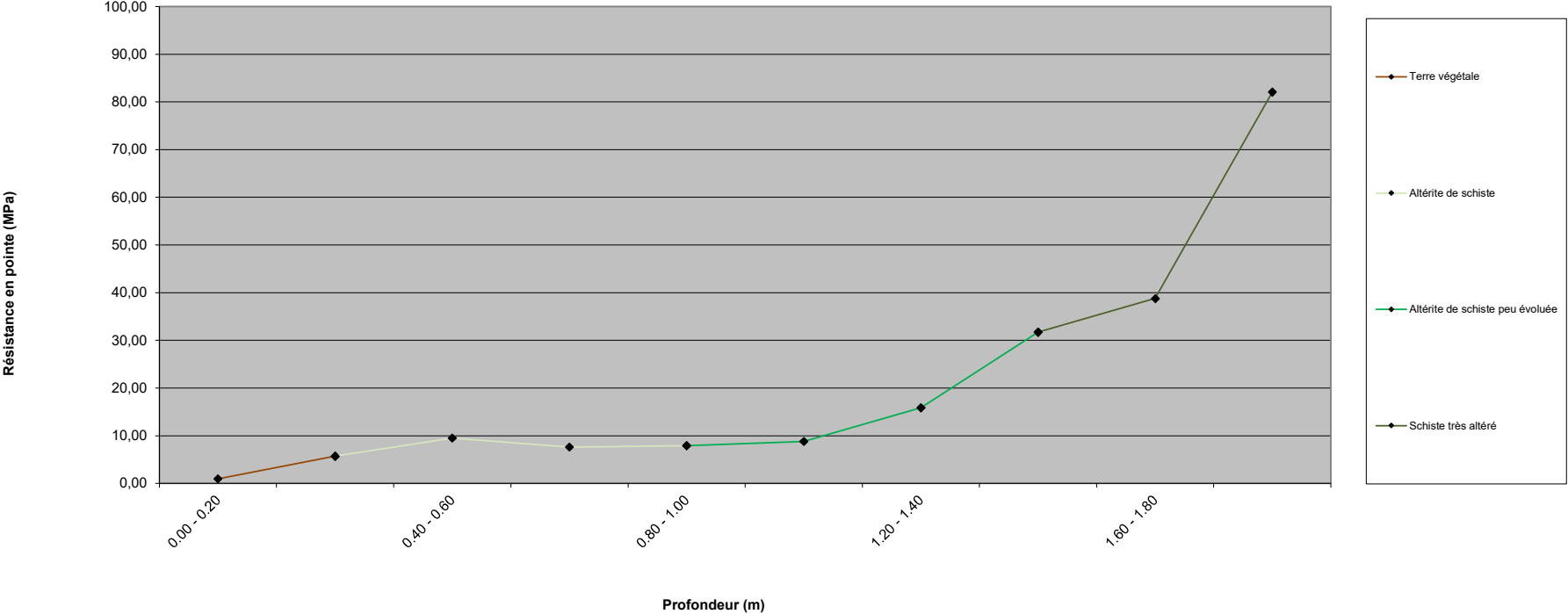
Sondage au pénétromètre dynamique - PD5 - cote NGF : 24,36 m
