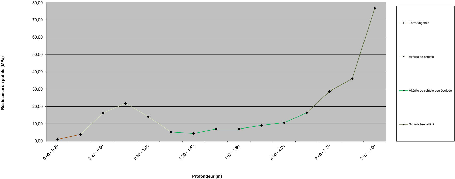
Sondage au pénétromètre dynamique - PD3 - cote NGF : 25,89 m
